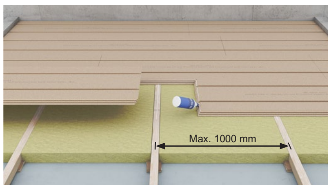
Figur 5 Klimagolv skarvas mellan regler. De läggs med förskjutning och utan skivskarvar i angränsande fack.
