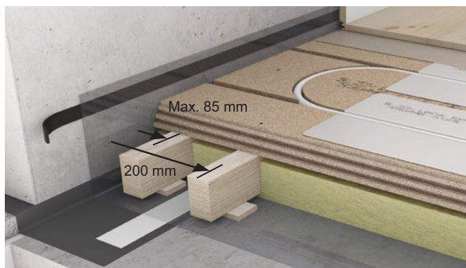
Figur 4 Klimagolv med kortling/kantregel max. 85 mm från vägg och extra regel under vändspåret. 200 mm från vägg.
